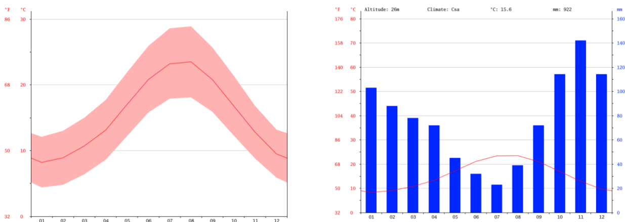
Figura 5-1-10 Grafico climatico Casavatore (Temperature mensili medie)
