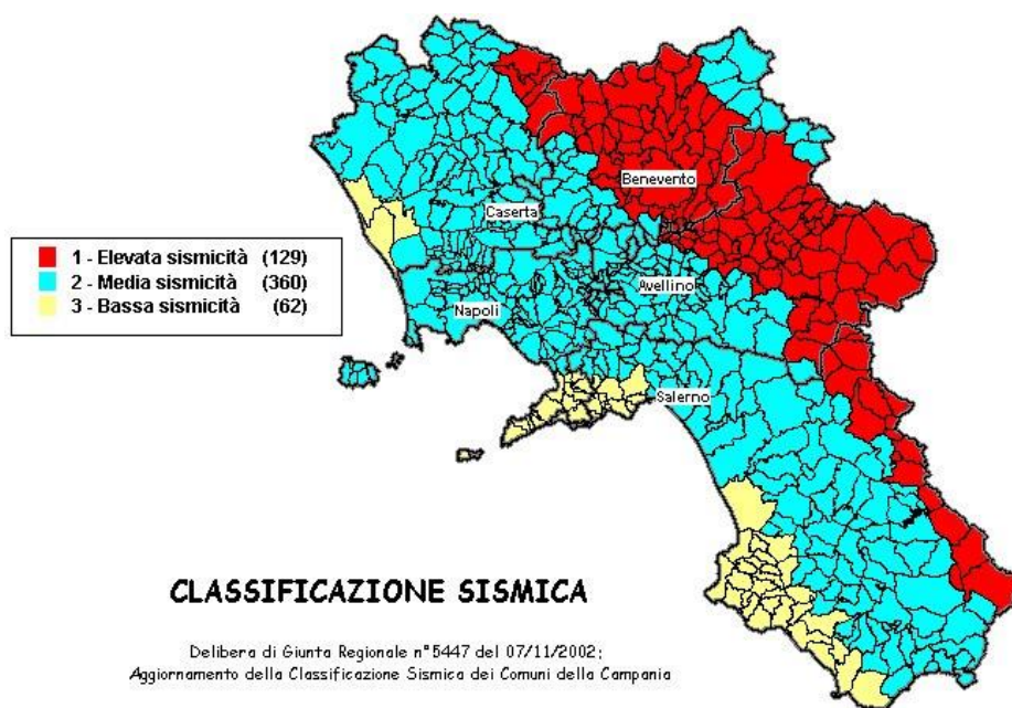
Figura 5-1-9 Classificazione sismica
